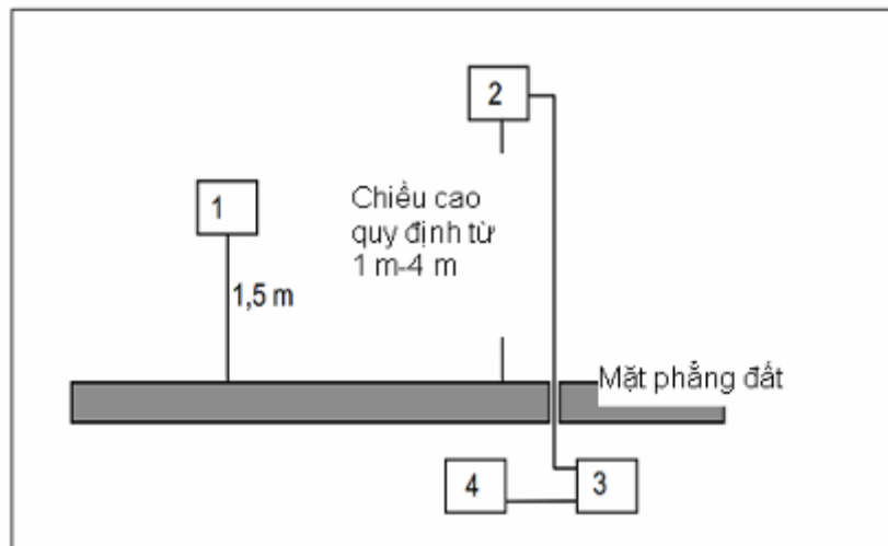
Hình B.1- Bố trí phép đo
